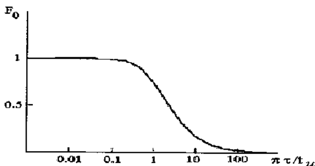
Пороговый характер максимальной силы отрыва дислокации
