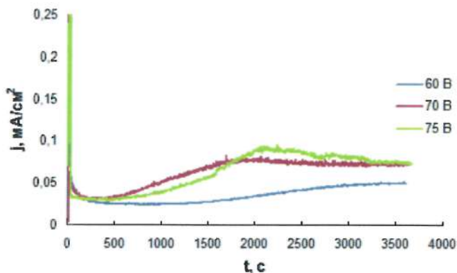
Рис. 1. Кривые j_a(t) , полученные при вольтстатическом анодировании в течение 1 ч образцов Nb в 1 \text{ M H}_2\text{SO}_4 + 1\% \text{ HF} при различных значениях напряжения U_a : 60, 70 и 75 В
