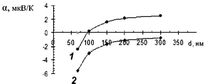
Рис. 1. Зависимости термоэлектрического коэффициента плёнок титана от толщины: 1 – относительно Рв, 2 – относительно Си
