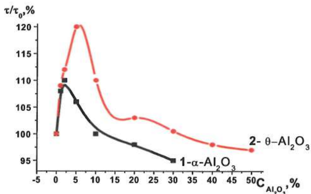
Рис. 2. Изменение сдвиговой прочности стальной проволоки к КМ на основе ЭД-22 с наполнителями: 1 – \alpha-Al_2O_3 ; 2 – \theta-Al_2O_3
