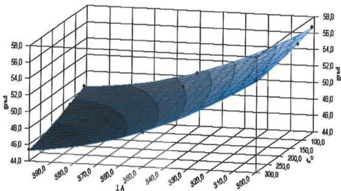
Рис. 2. Зависимость краевого угла смачивания покрытия на основе порошка ГА от тока дуги и продолжительности пропитки
