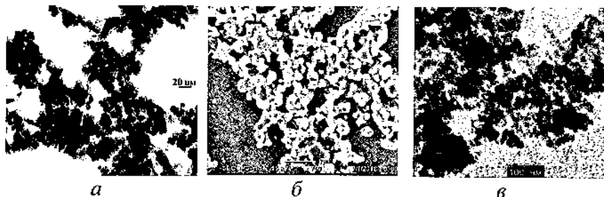
Рис. 1. ПЭМ изображение композита (\text{ГА})\text{Fe}_3\text{O}_4 (а), СЭМ изображение (б) и (\text{ГА})\text{Fe}_3\text{O}_4 ПАД-С5 (в), \times 100000 раз
