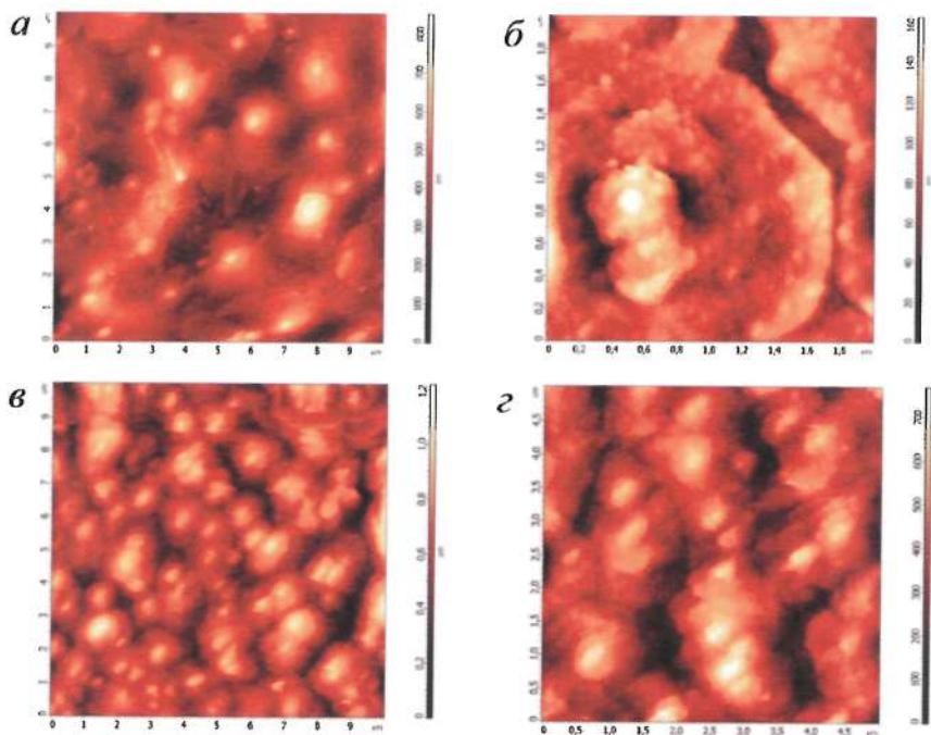
Рис. 3. АСМ-изображения поверхности СП Nb, анодированного в 1 М \text{H}_2\text{SO}_4 + 1% HF при напряжении U_a = 60 В в течение 1 ч (а, б) и 2 ч (в, з)
