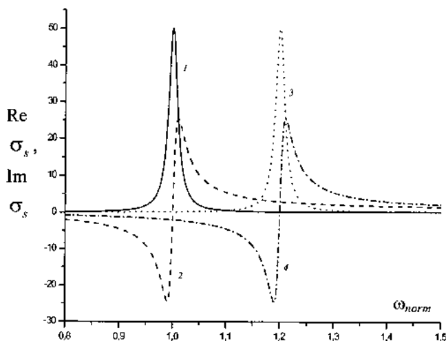
Рис. 1. Частотная зависимость действительных (кривые 1, 3) и мнимых (кривые 2, 4) частей проводимостей метаповерхности на основе одноосной плазменной решетки [2]: продольной (кривые 1, 2) и поперечной (кривые 3, 4)
