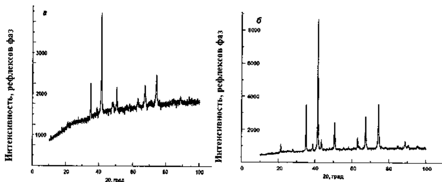
Рис. 1. Рентгенофазовый анализ: a – (\text{Mn,Zn})\text{Fe}_2\text{O}_4 (1); б – (\text{Ni,Zn,Cu})\text{Fe}_2\text{O}_4 (2)
