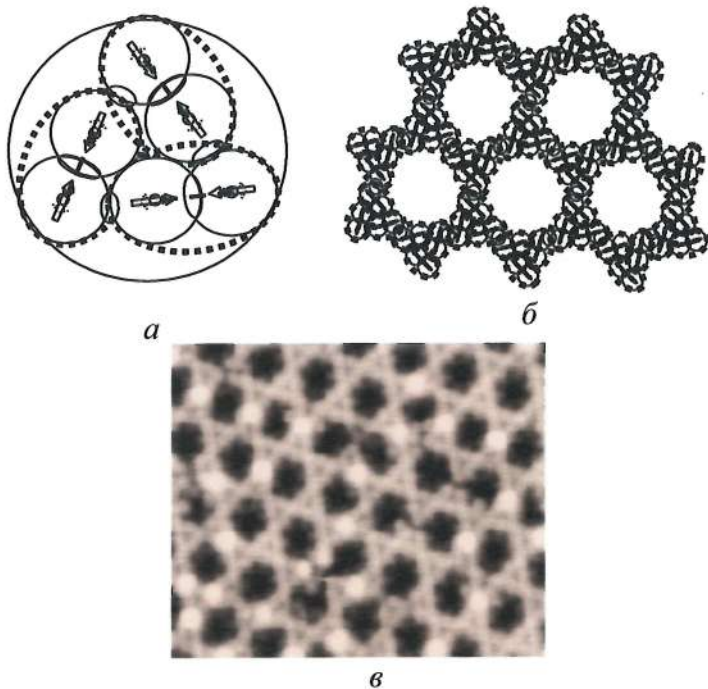
Рис. 3. Кластеры индия, полученные методом расчета и экспериментально на СТМ: а – кластер индия на поверхности кремния; б – кластерная решеточная структура индия на поверхности кремния; в – кластерная решеточная структура индия на поверхности кремния (эксперимент)
