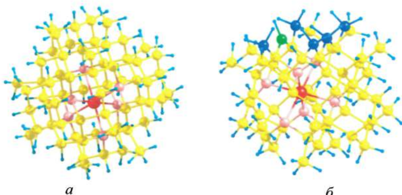
Рис. 1. Структуры кластеров: a – «объемный» C_{69}[GeV]H_{84} ; б – «поверхностный» C_{64}[GeV]H_{68}(100)_{H11} , оптимизированных методом DFT/UKS/PW91/RI/def2-SVP. Обозначения атомов: С – желтый, Ge – красный, С ближайшие соседи к атому Ge – розовый, поверхностные С – темно-синий, с обрванными связями – зеленый, H – синий
