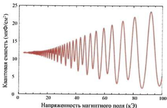
Рис. 2. Зависимость квантовой емкости от напряженности магнитного поля при \Gamma = 0.3 мэВ, \epsilon_F = 0.03 эВ, \Delta_h = 4 мэВ, n_e = 4 \cdot 10^{15} м -2 , v = 3 \cdot 10^5 м/с
