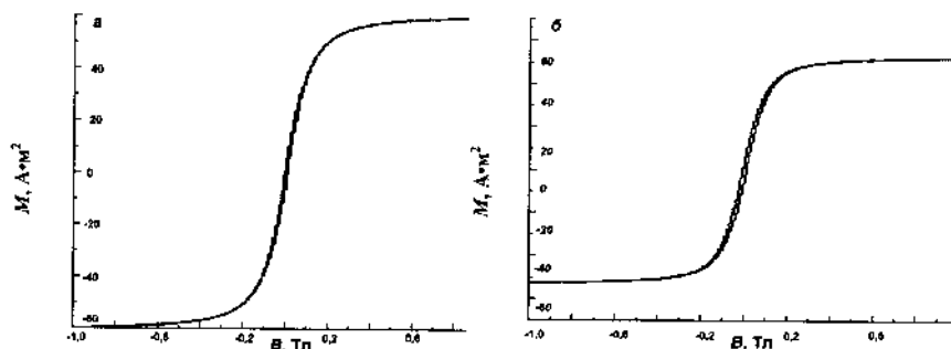
Рис. 2. Кривые намагниченности порошков ферритов: a (\text{Mn,Zn})\text{Fe}_2\text{O}_4 (1); б (\text{Ni,Zn,Cu})\text{Fe}_2\text{O}_4 (2) при 300 К
