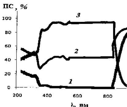
Рис. 3. Спектры пропускания (1, 2) и поляризующая способность (ПС) (3) ПВС-пленок, содержащих смесь красителей Chicago Sky Blue , \text{M}_3\text{H} и \text{IR-3} и композит \text{Fe}_3\text{O}_4\text{-Au}
