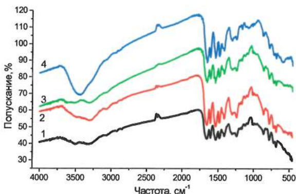
Рис. 4. ИК спектры образцов фенилона С2 (1) и с добавками 17мас.% \gamma (2), \theta (3), \alpha - \text{Al}_2\text{O}_3 (4)
