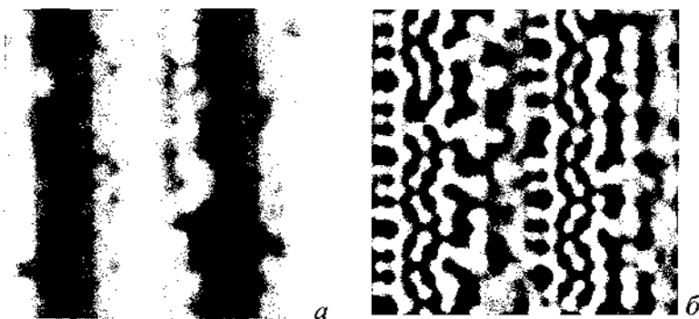
Рис. 6. Vicинальная поверхность кремния (557): а – изображение, полученное на СТМ; б – изображение vicинальной поверхности кремния [7]
