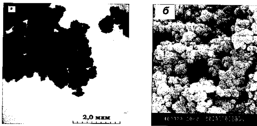
Рис. 3. Изображения порошков ферритов: a – (\text{Mn,Zn})\text{Fe}_2\text{O}_4 (1) (ПЭМ); б – (\text{Ni,Zn,Cu})\text{Fe}_2\text{O}_4 (2) (СЭМ)
