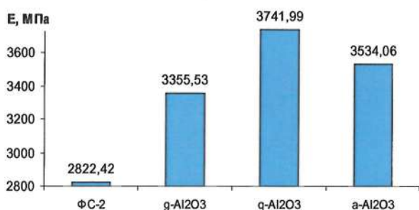
Рис. 5. Разрушение матрицы С2 (1), КМ (2), модуль упругости С2 и КМ с \gamma -, \theta -, \alpha - Al 2 O 3 (3)
