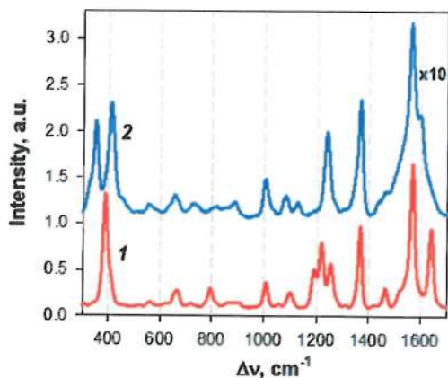
Рис. 2. Спектры ГКР CuTMруP4 (1) и CuTSPР4 (2) на плазмонной пленке из нанокompозита (ГА)Ag, синтезированного по методике (II)
