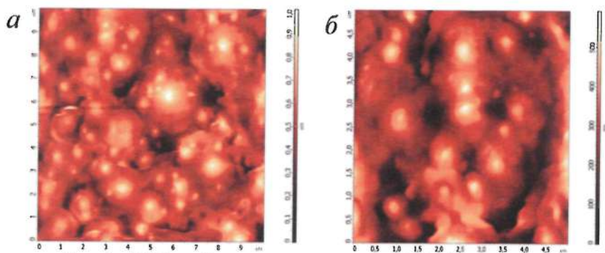
Рис. 4. АСМ-изображения поверхности СП Nb, анодированного в 1 М \text{H}_2\text{SO}_4 + 1% HF при напряжении U_a = 70 В в течение 1 ч
