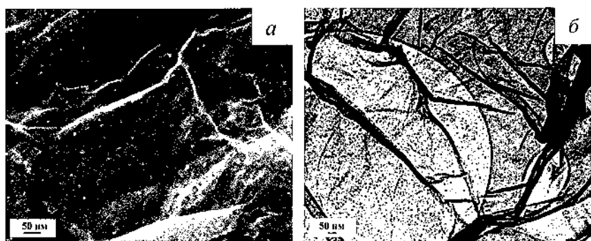
Рис. 1. Микрофотографии СЭМ (а) и ПЭМ (б) композита Ni/GPM
