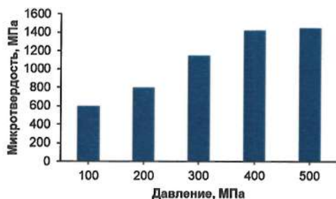
Рис. 1. Зависимость микротвердости покрытий на основе порошковых систем медь–УНТ от давления электродов
