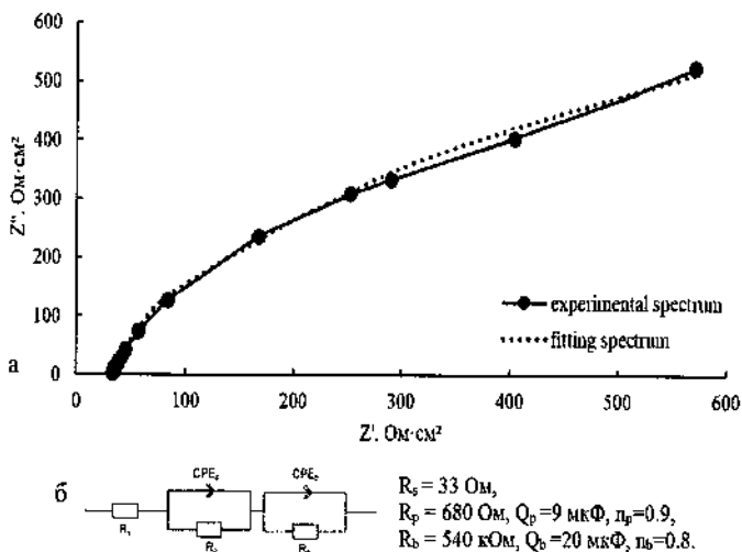
Рис. 3. Экспериментальная и модельная диаграммы Найквиста, Z''(Z') , для анодированного в 1M H_2SO_4 + 1%HF Nb (а); (б) эквивалентная электрическая схема и значения элементов ЭЭС ( Q_p и Q_b – значения элементов CPE_p и CPE_b )
