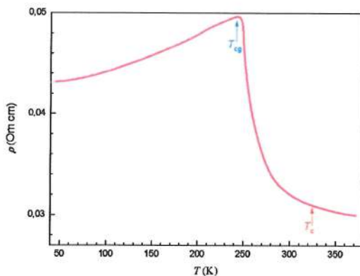
Рис. 2. Температурная зависимость электросопротивления нанокompозита Cd_3As_2 + 44.7\% MnAs в интервале температур 40–380 К. Критическая температура кластерного стекла T_{cg} = 241 К, точка Кюри T_C = 325 К
