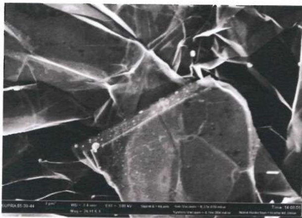
Рис. 9. Характерный вид топологии наноструктурированного абсорбера из многослойного графена на диэлектрической подложке
