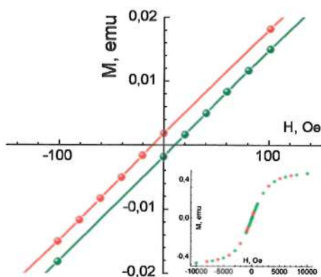
Рис. 4. Участок изотермической петли гистерезиса намагниченности \text{Cd}_3\text{As}_2+44.7\% \text{MnAs} при 300 К, демонстрирующий небольшую величину коэрцитивной силы (10 Э). Во вставке петля намагниченности – ввиду малости гистерезиса незаметен. Зеленые точки сняты при росте магнитного поля, красные при сбавлении
