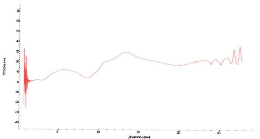
Рис. 8. Спектр отражения оптического излучения тестового чувствительного элемента датчика теплового потока с поглощающим покрытием (0,57 в диапазоне 0,1–14,0 мкм)
