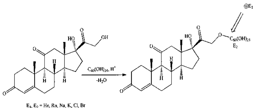
Рис. 1. Схема построения эндоэдрических (@) фуллерено-локортизоновых кластеров (E 1 )@C 60 (OH) 23 OC 21 H 27 O 5 (E 2 )
