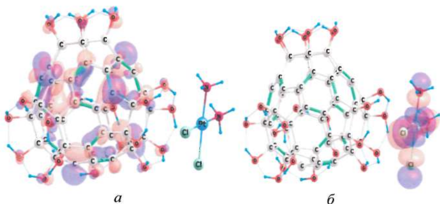
Рис. 5. Локализация: а – ВЗМО, б – НСМО комплекса C_{60}(OH)_{24} + Cis после расчета методом DFT с учетом растворителя (воды)
