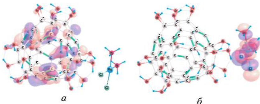
Рис. 4. Локализация: а – ВЗМО, б – НСМО комплекса C_{60}(OH)_{24} + Cis после расчета методом DFT в безводной среде
