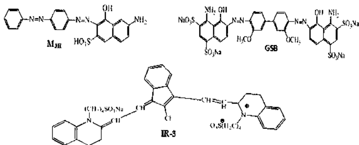
Рис. 1. Структуры красителей
