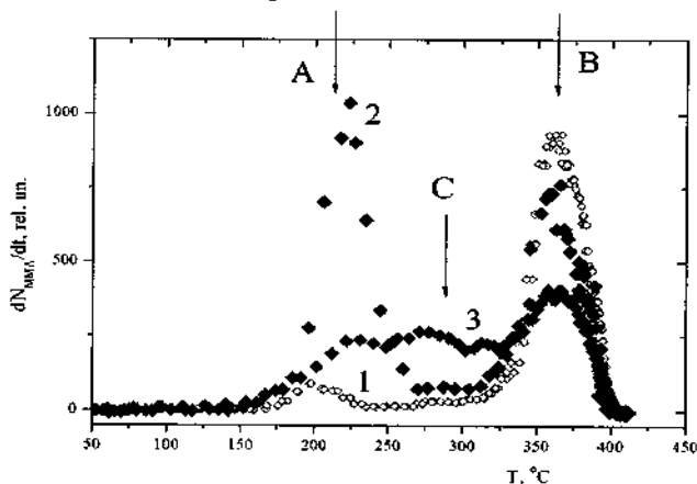
Рис. 1. ТДМС мономера MMA в координатах скорость десорбции-температура при нагревании пленок чистого ПММА без облучения (1), чистого ПММА после УФ облучения в течение 5 минут (2), композита ПММА-С 60 с концентрацией С 60 ~8 мас.% после 5 мин УФ облучения (3)
