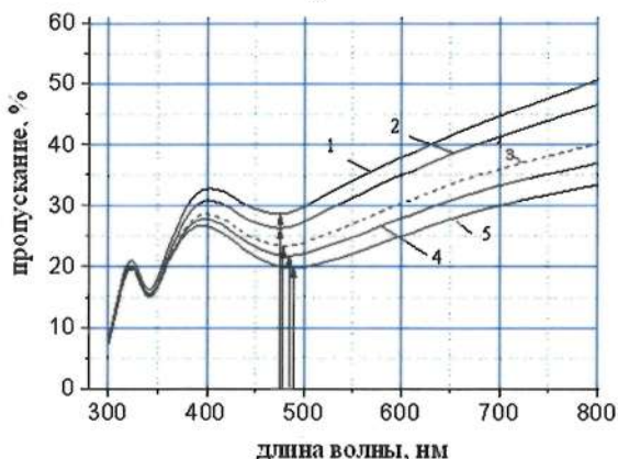
Рис. 4. Спектры пропускания нанокompозитов Ag-C 60 с различными ППМ компонентами: a – Ag: (1–6) ~ (0.85–1.9)·10 -6 г/см 2 ; C 60 : (1–6) ~ (6.5–3.4)·10 -7 г/см 2 ; б – Ag: (1–5) – (6.0;6.4;7.0;7.4;8.0)·10 -6 г/см 2 ; C 60 : (1–5) – 2·10 -6 г/см 2
